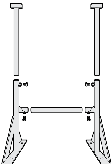
4 x skruv 2 x fot 2 x top 1 x distans
