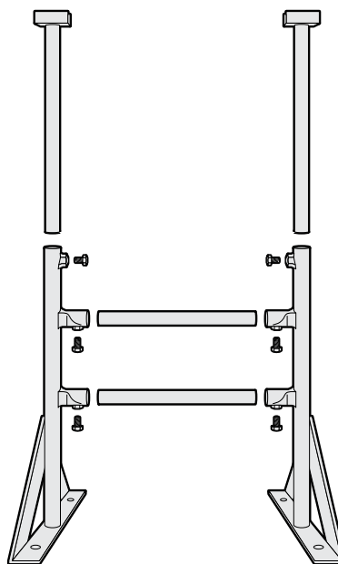
6 x skruv 2 x fot 2 x top 2 x distans
