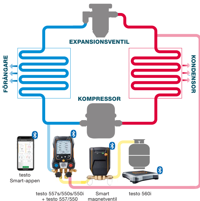
Schematiskt diagram för automatisk köldmediefyllning
